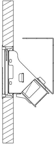
Vista in sezione B-B Scala: 1:2
